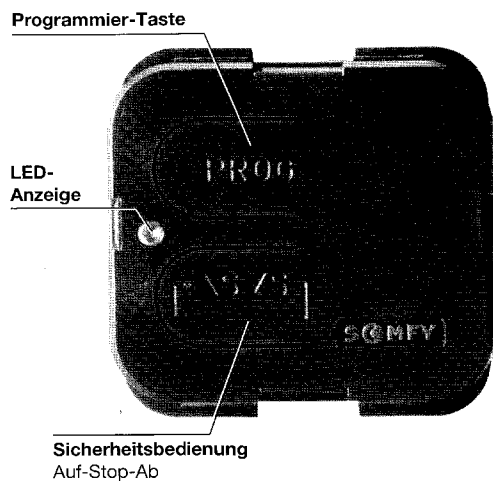
Motormodul RCE 800/RCE 801
